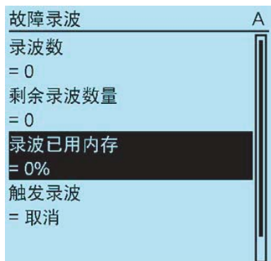
图50: 通过LHM I/O人机界面监视故障录波
