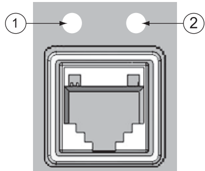
图 5: RJ-45 通讯端口和LED指示灯
